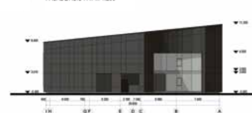
FASĀDE ASIS 1-A / M 1:200
