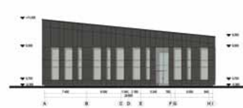
FASĀDE ASIS A-I / M 1:200
